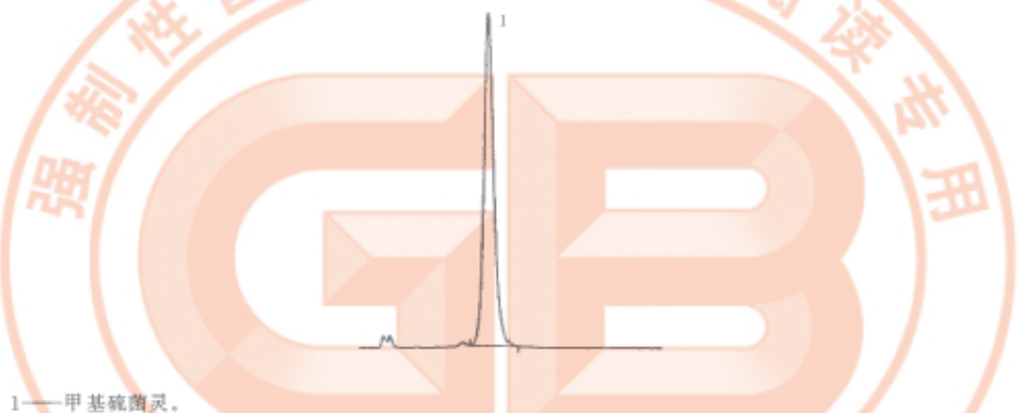
图 1 甲基硫菌灵可湿性粉剂的高效液相色谱图
