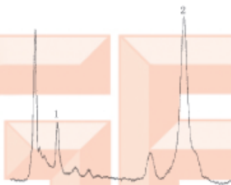
图2 HAP和DAP标样的液相色谱图
